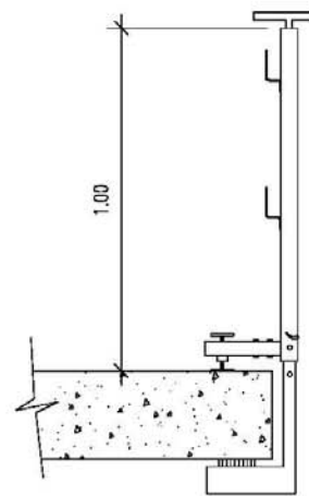
SOPORTE " TIPO - 1 "
