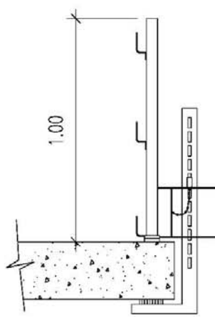
SOPORTE " TIPO - 2 "
