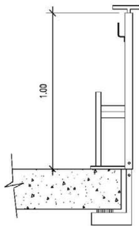
SOPORTE " TIPO - 3 "
